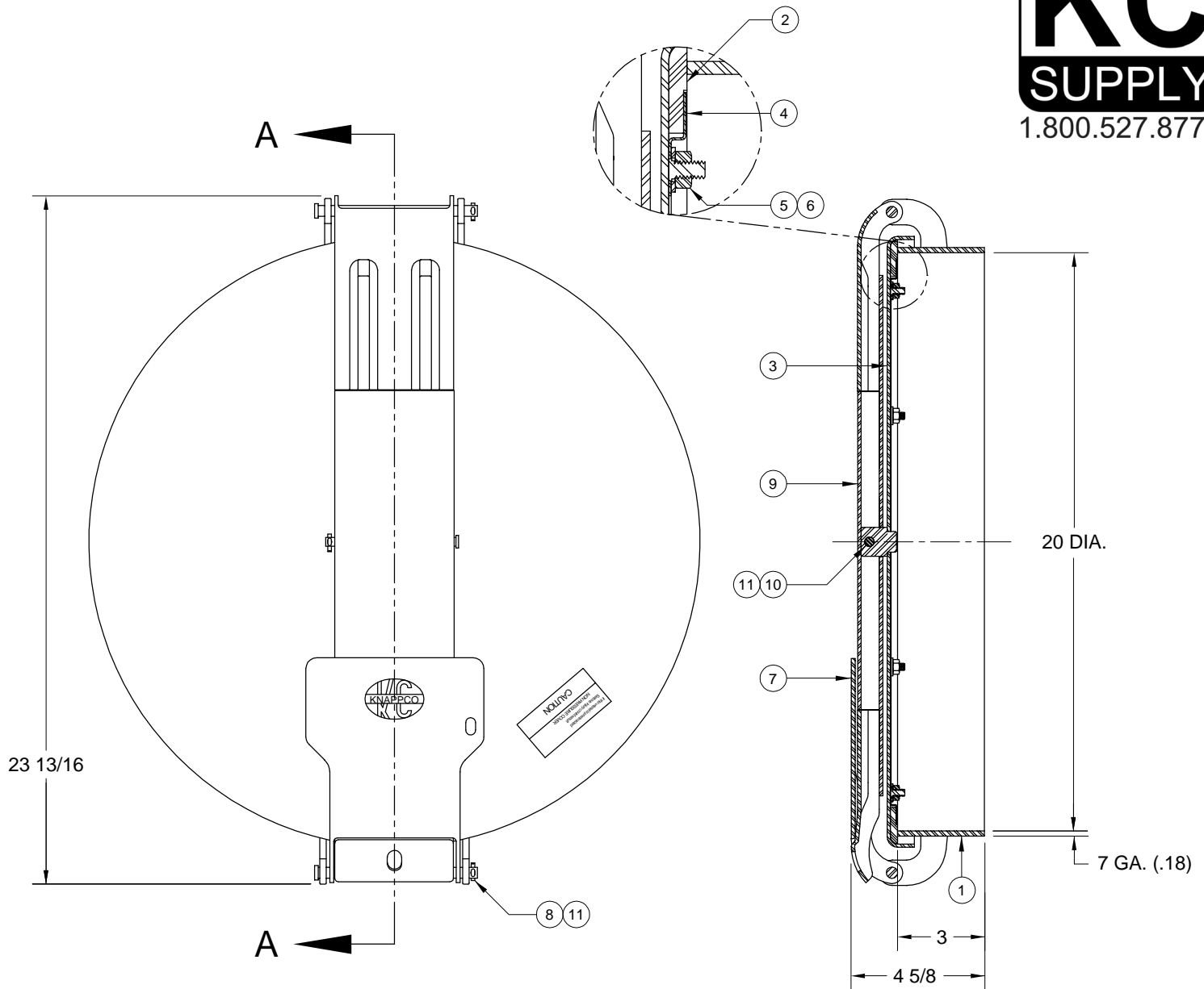
SECTION A-A
