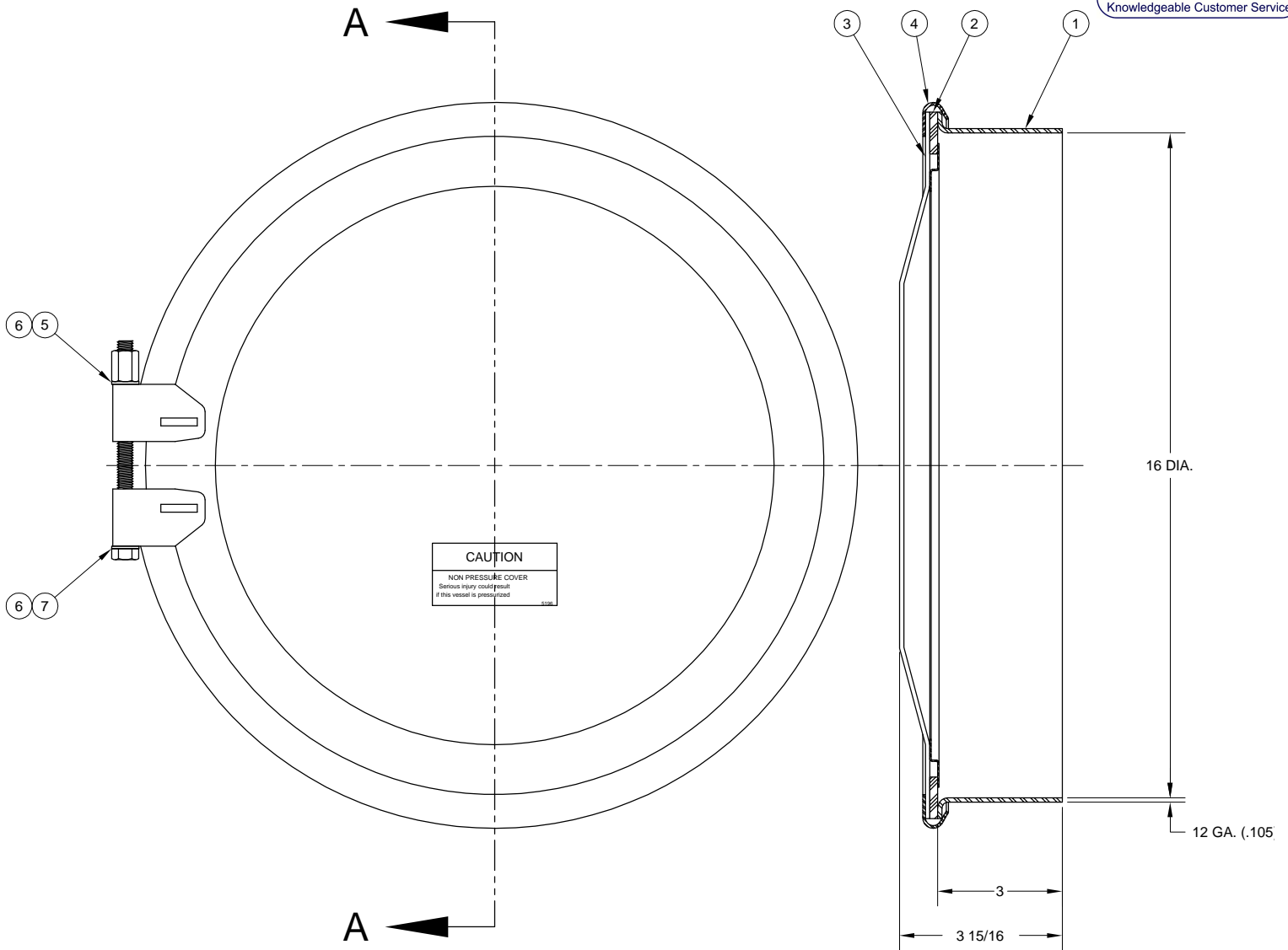
SECTION A-A
